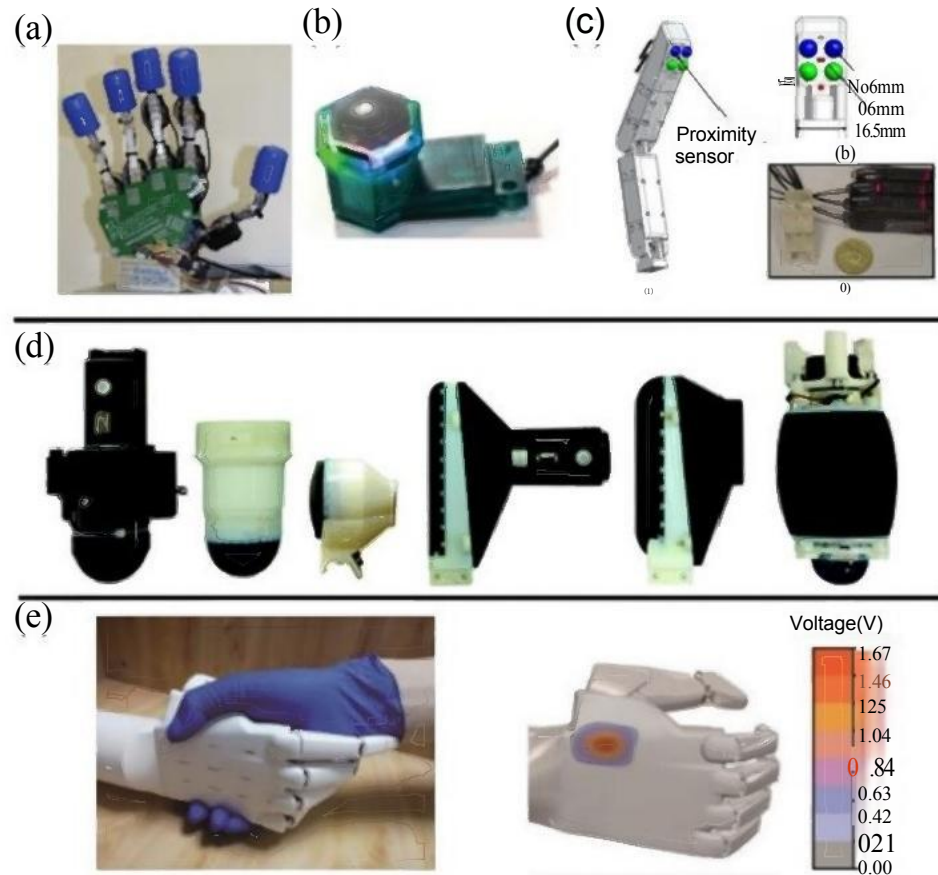
图表 28：灵巧手外部传感器分布情况
