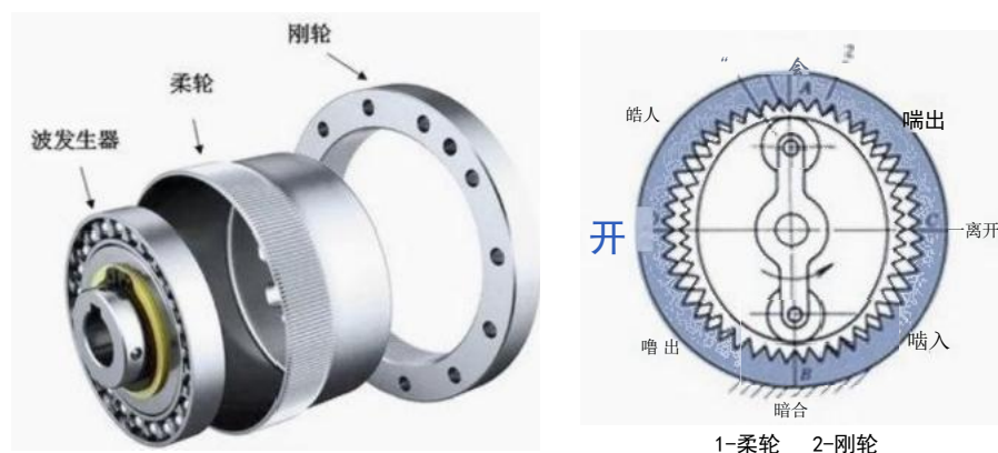
图 2.0：谐波减速器结构示意图
